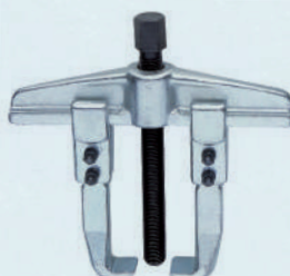
Art. 00903 Estrattori forgiati scorrevoli su guide a 2 griffe Per meccanica - In acciaio forgiato verniciato Griffe reversibili per uso esterno ed interno
