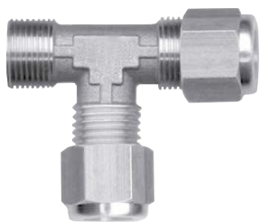
RACCORDO A "T" LATERALE CONICO MASCHIO / SEITLICHER T-ANSCHLUSS, KONISCH, MIT AUSSENGEWINDE / SIDE CONICAL MALE "T" CONNECTOR / RACCORD EN "T" LATÉRAL CONIQUE MÂLE / TE LATERAL CÓNICO MACHO
